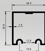
PERFIL CONCAVO PANTOGRÁFICO
